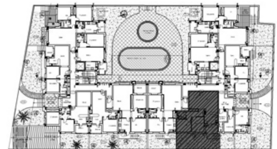
PLAN RDC
